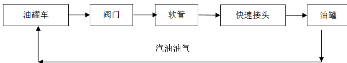
图 2-3 汽油卸油工艺流程框图
