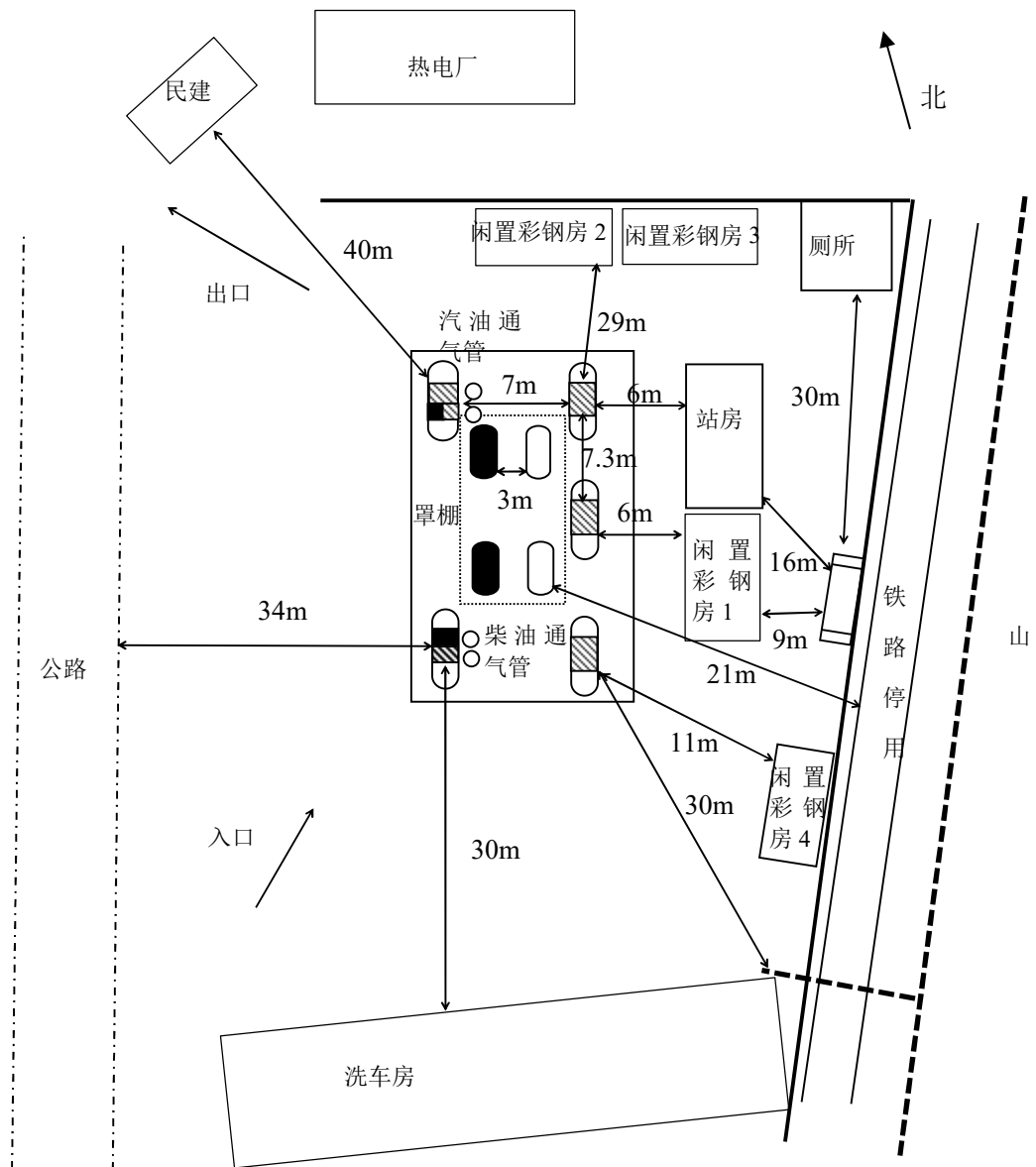
图 2-2 加油站总平面布置图
