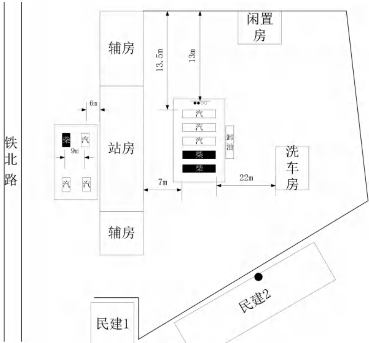
图2.3-3 总平面布置示意图
