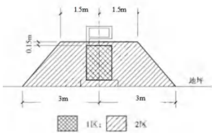
附图 1 车用乙醇汽油加油机爆炸危险区域划分
