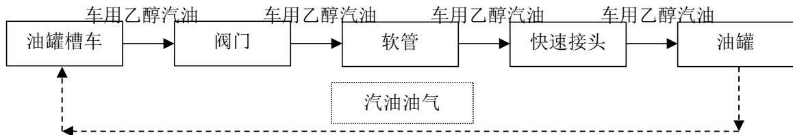
图2.4-1 车用乙醇汽油卸油工艺流程框图
