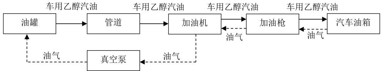
图2.4-3 车用乙醇汽油加油工艺流程框图
